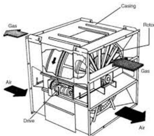
عکس Regenerator - حالت عمودی
